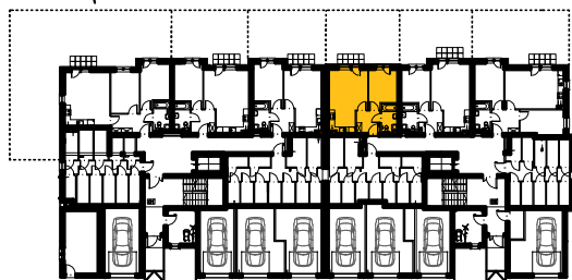
RZUT PARTERU
